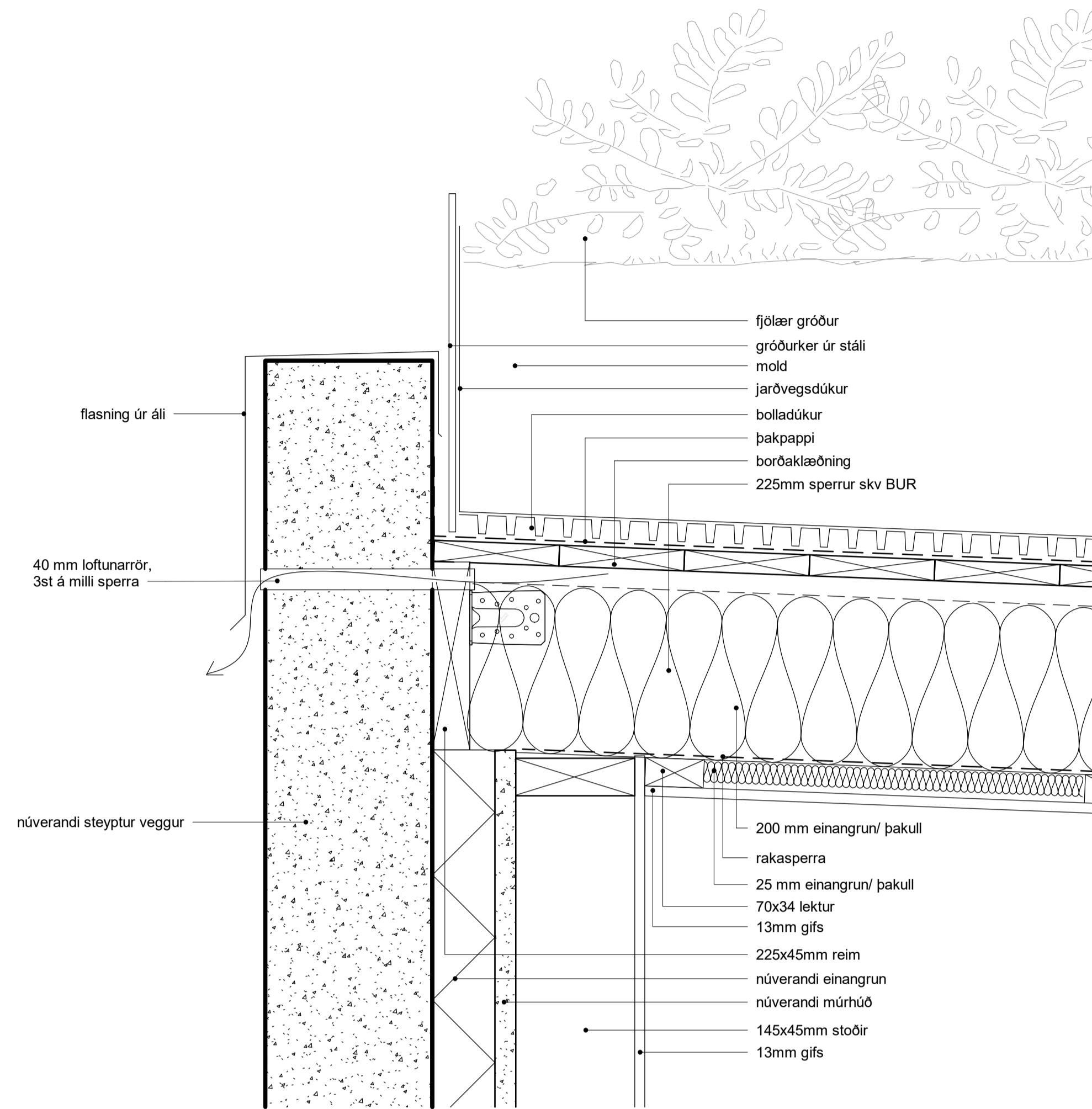
1 Deili - útveggur/ þak 1 : 5
