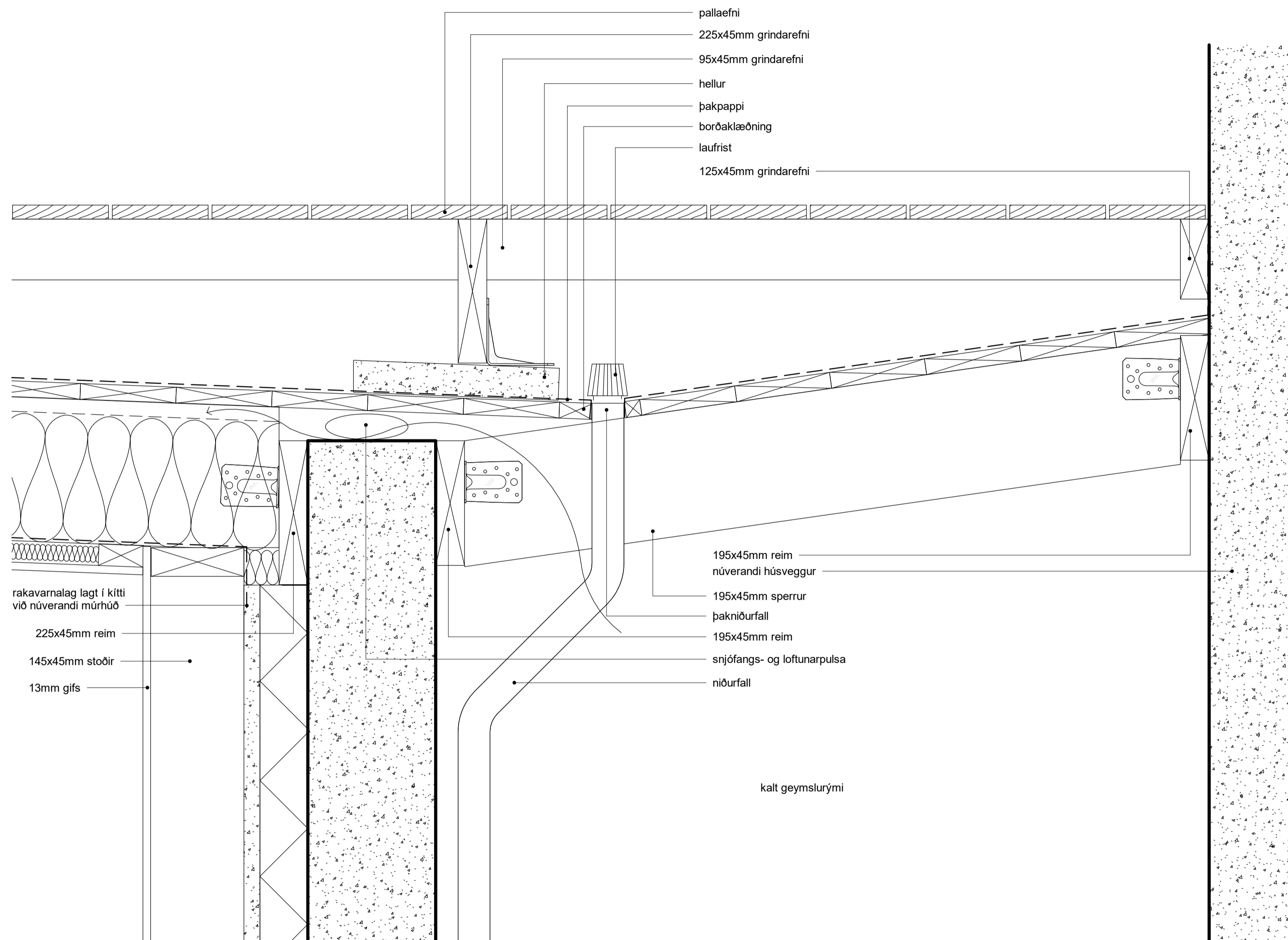
2 Deili - þak/ geymsla 1 : 5
